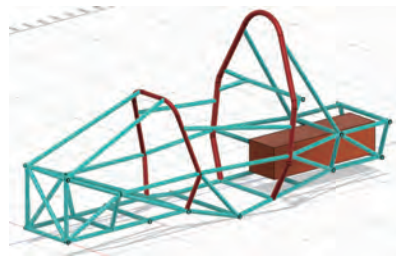
車体構造の等価構造設計中の様子
