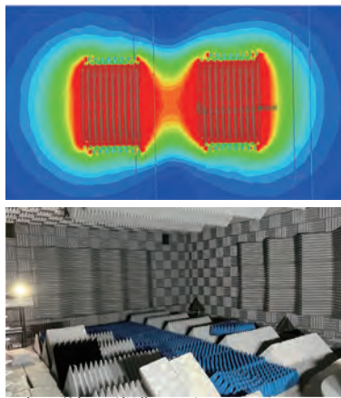
(上)電波の可視化 (下)シールドルーム
